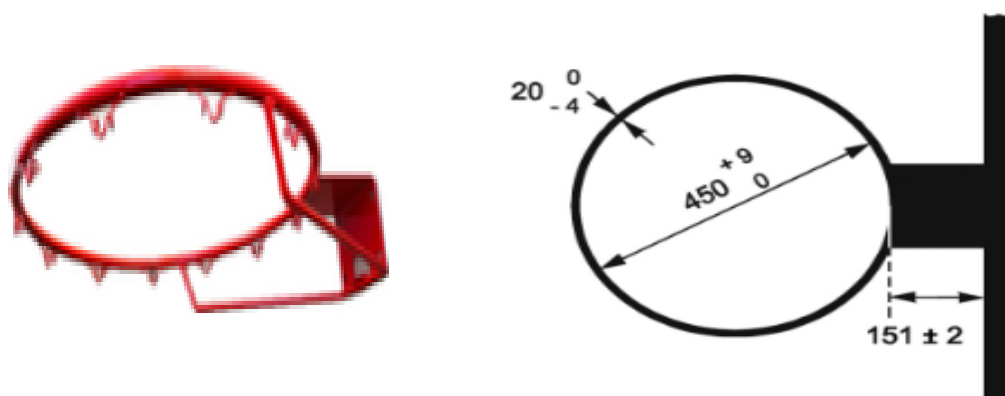
Рис. 13.4. Кільце
