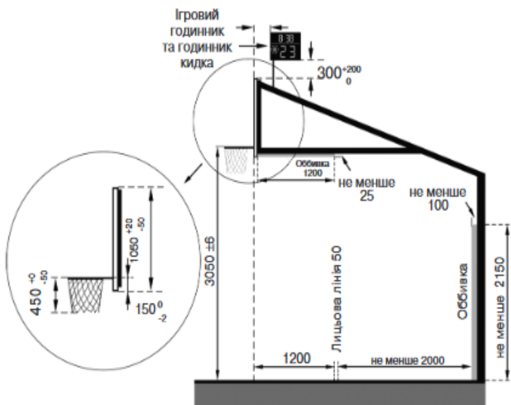
Рис. 13.2. Конструкція щита
