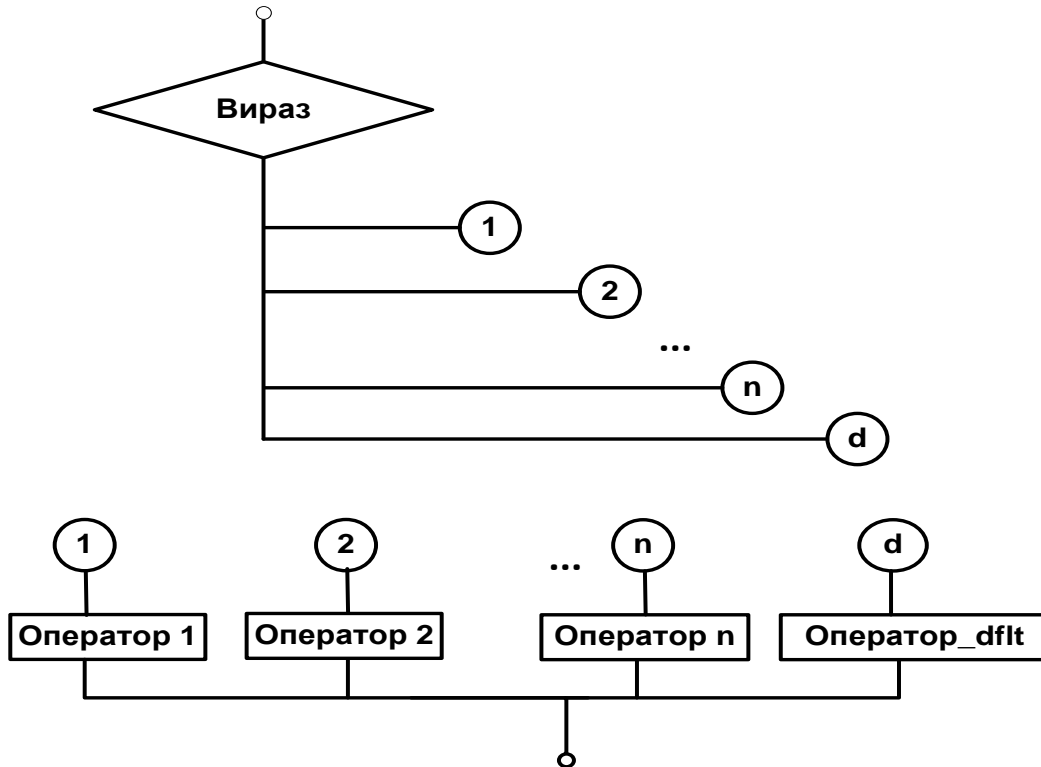
Рис. 13. Графічна схема оператора switch
