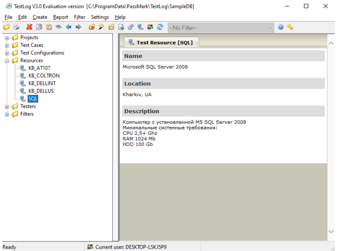
Рис. 13 Сутність Resources
