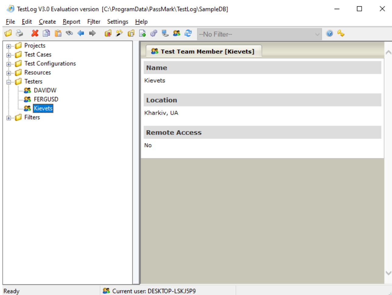
Рис. 11 Сутність Tester
