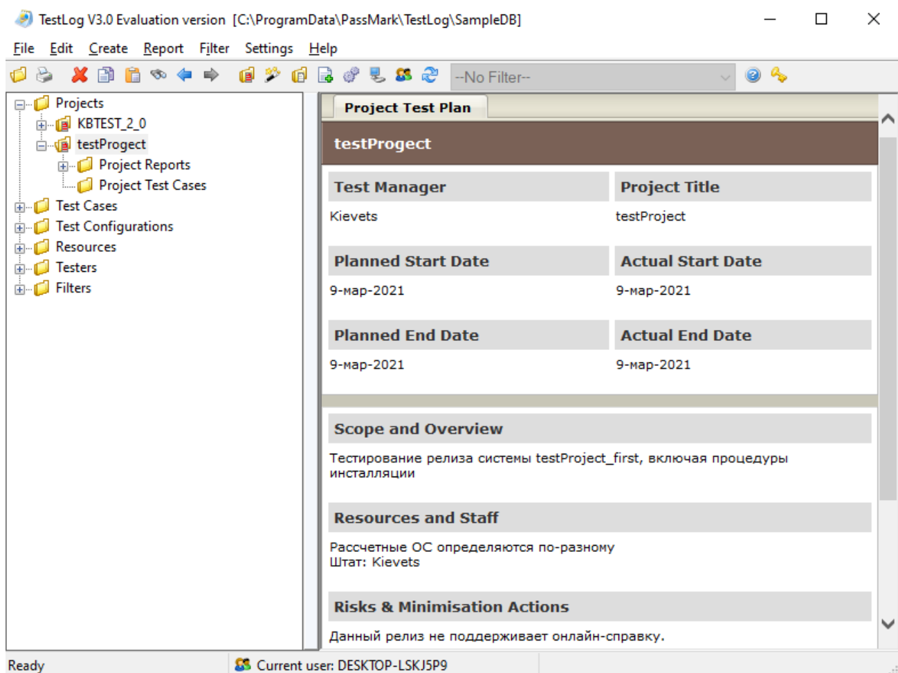
Рис. 10 Сутьность Project
