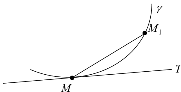
Рисунок 2 – Дотична T до кривої \gamma в точці M
